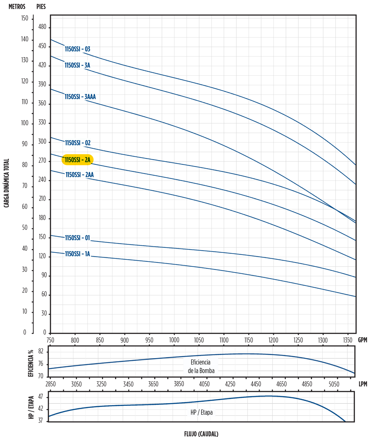
CURVA DE RENDIMIENTO - SSI 10" 1150 GPM - 01-03 ETAPAS
