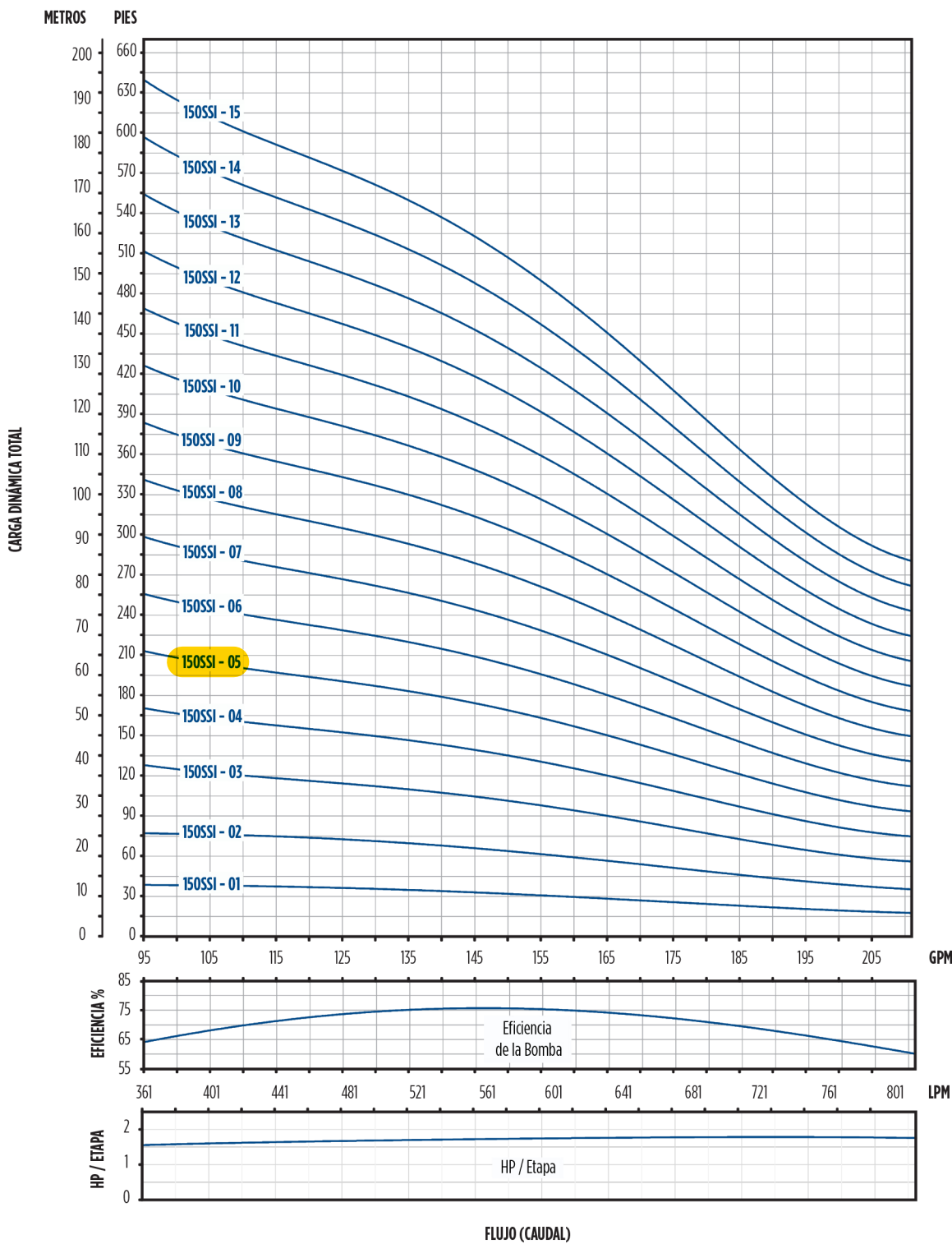
CURVA DE RENDIMIENTO - SSI 6" 150 GPM - 01-15 ETAPAS
