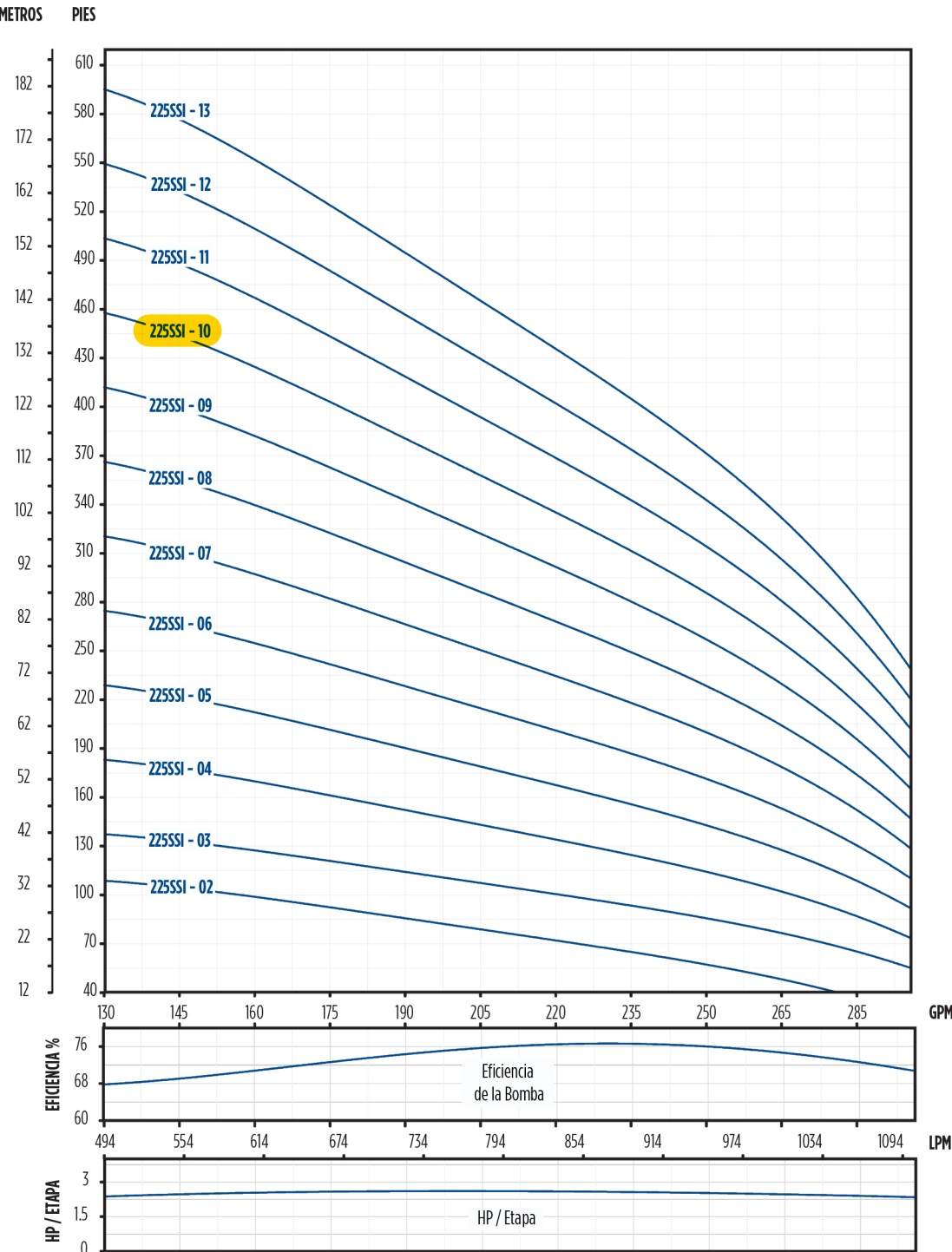
CURVA DE RENDIMIENTO - SSI 6" 225 GPM - 02-13 ETAPAS
