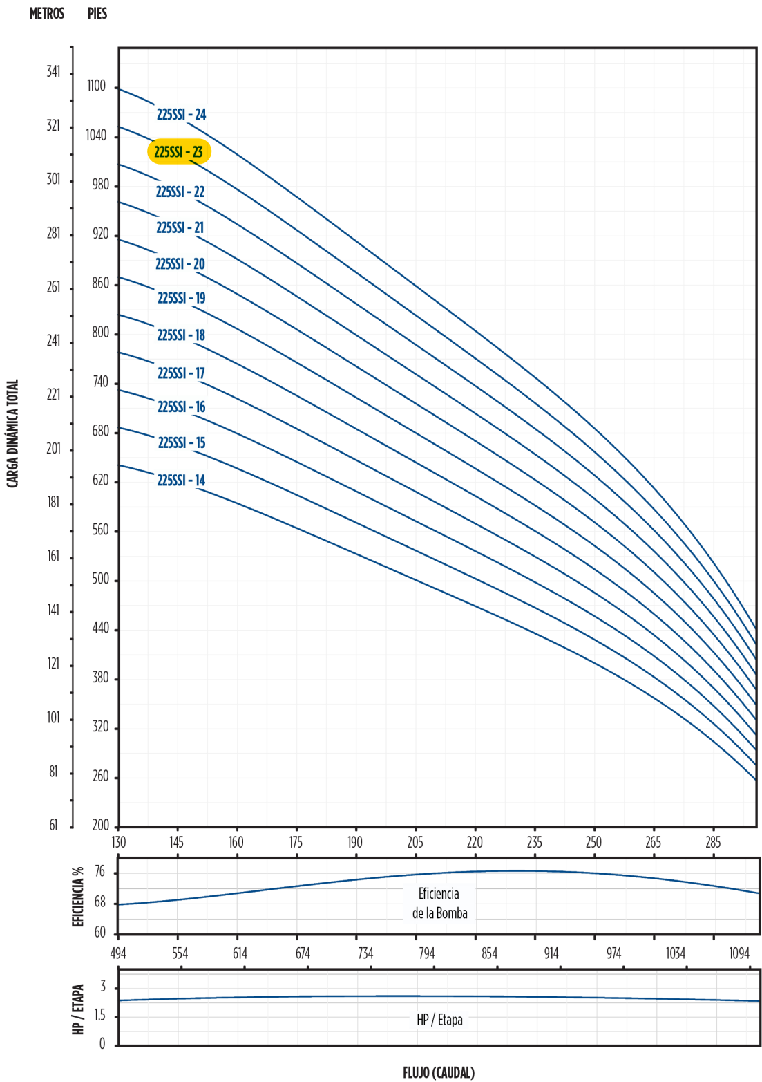
CURVA DE RENDIMIENTO - SSI 6" 225 GPM - 14-24 ETAPAS
