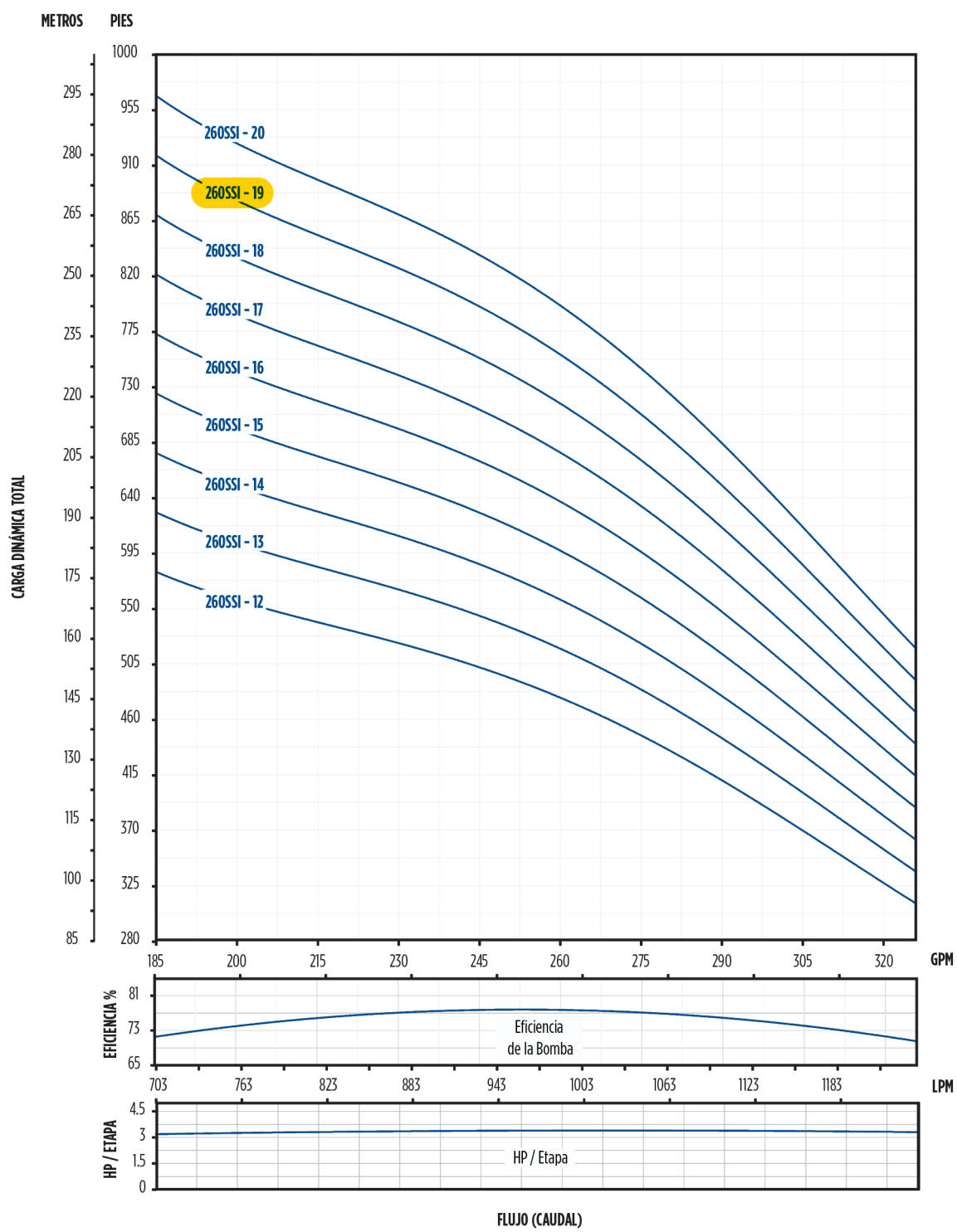
CURVA DE RENDIMIENTO - SSI 6" 260 GPM - 12-20 ETAPAS
