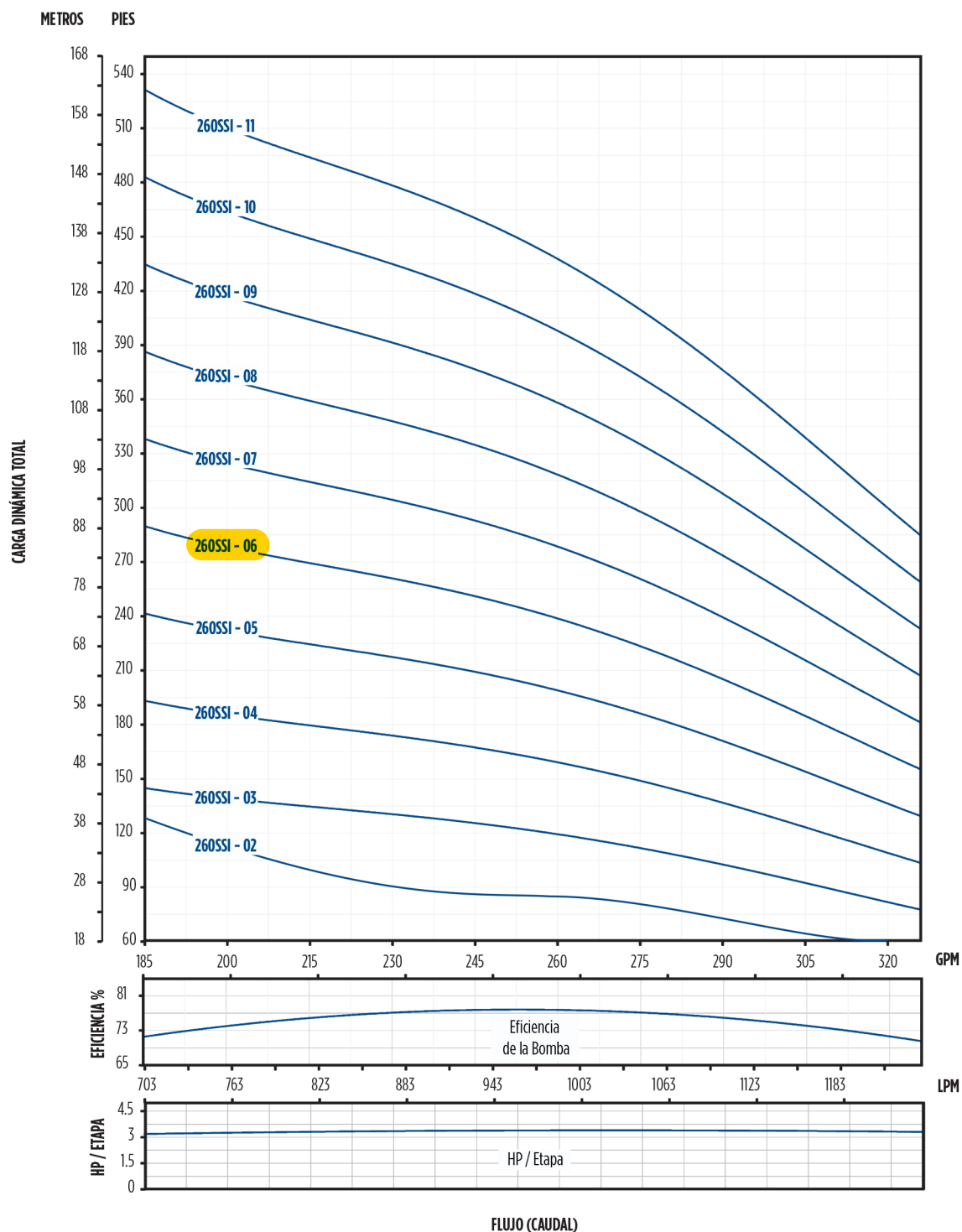
CURVA DE RENDIMIENTO - SSI 6" 260 GPM - 02-11 ETAPAS
