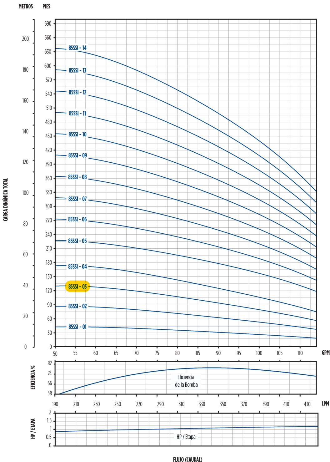
CURVA DE RENDIMIENTO - SSI 6" 85 GPM - 01-14 ETAPAS
