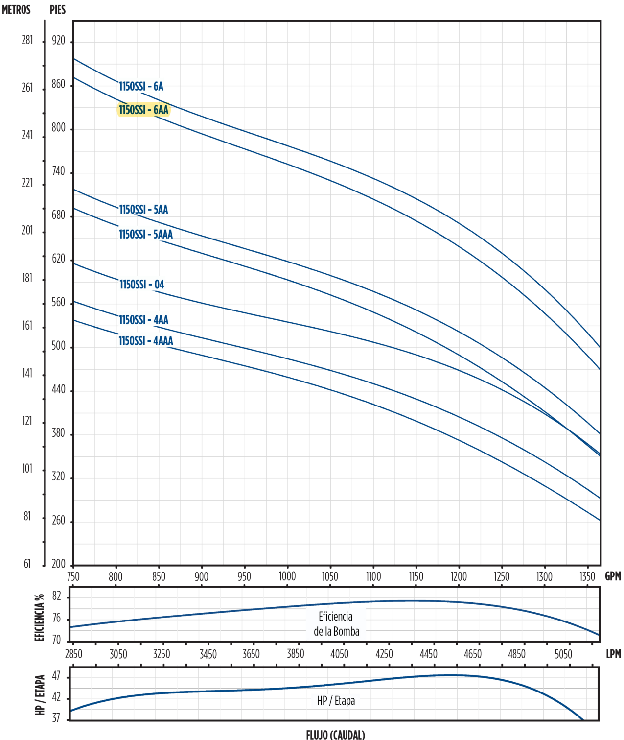
CURVA DE RENDIMIENTO - SSI 10" 1150 GPM - 04-06 ETAPAS
